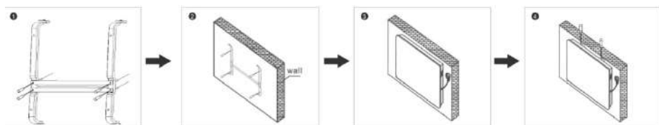
Рис. 2 Установка на стену
