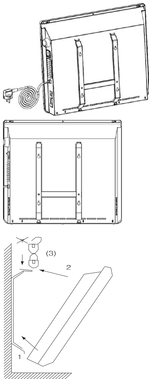
Рис.5. Настенная установка
