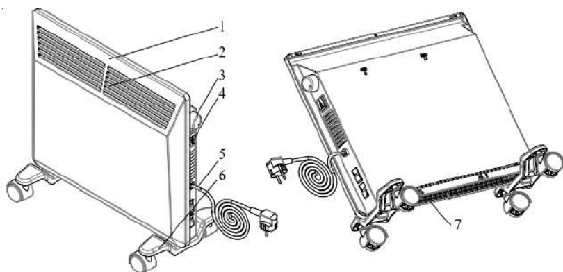
Рис.1 Устройство конвектора
